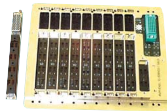
10 バックプレーンMT 角型コネクタにMTフェルールを組込み、 特殊なラック型シェルに取付
