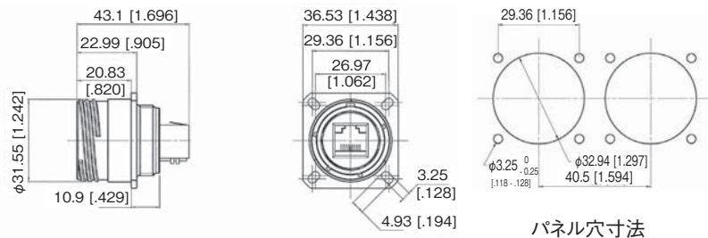
パネル穴寸法
