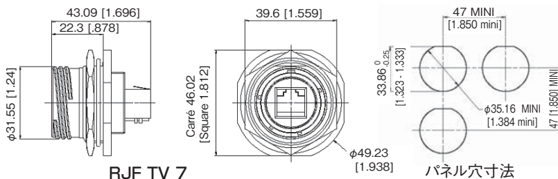
パネル穴寸法
